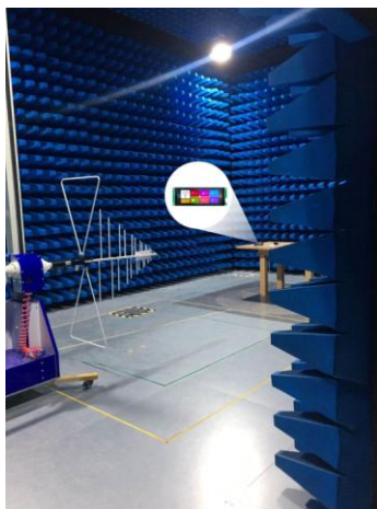
图 4-4 RE 测试图
