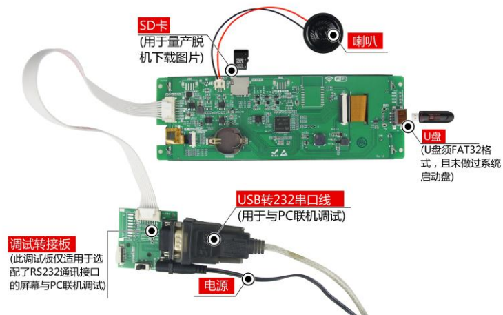
图 1-4 RS232 调试工具图
