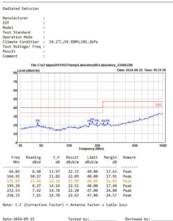
图 4-5 RE 测试水平方向
