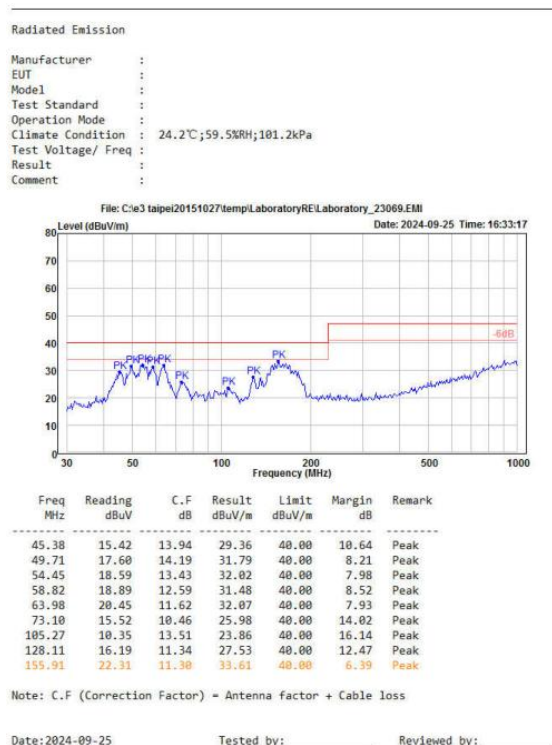
图 4-6 RE 测试垂直方向
